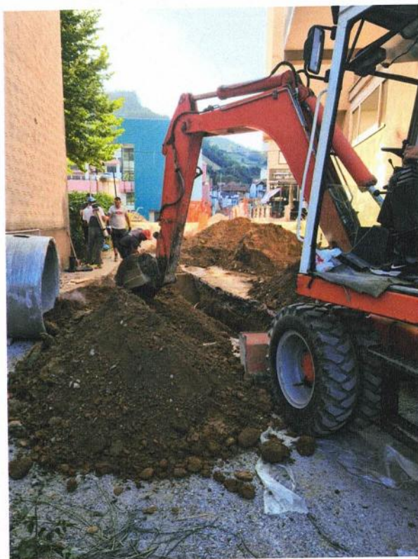
Slike: Izvođenje radova na izradi fekalne kanalizacije PVC DN 250 mm za potrebe OŠ „Dušan Korać“ u ul. Voja lješnjaka
