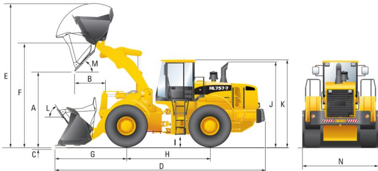
Slika 39. Konstruktivne karakteristike utovarača HYUNDAI HL757/7
