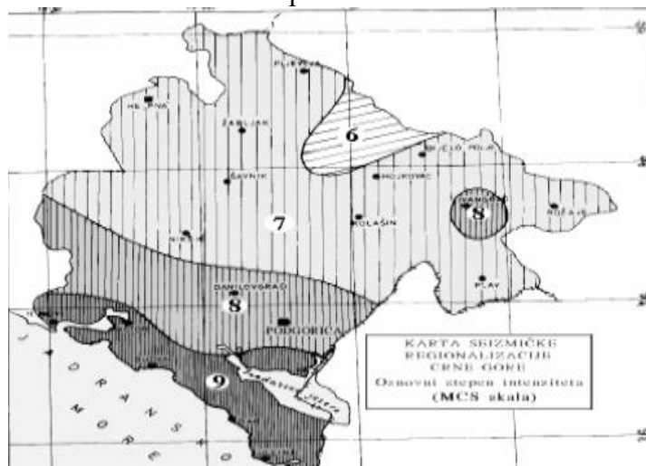
Slika 18. Karta seizmičke rejonizacije teritorije Crne Gore sa granicom opštine Bijelo Polje
