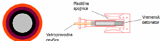
Slika 30. Poprečni presjek Nonel vatroprovodne cijevčice i izgled Nonel konektora
