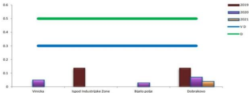
Slika. 42. Sadržaj ortofosfata(fosfata) u rijeci Lim (mg/l)
