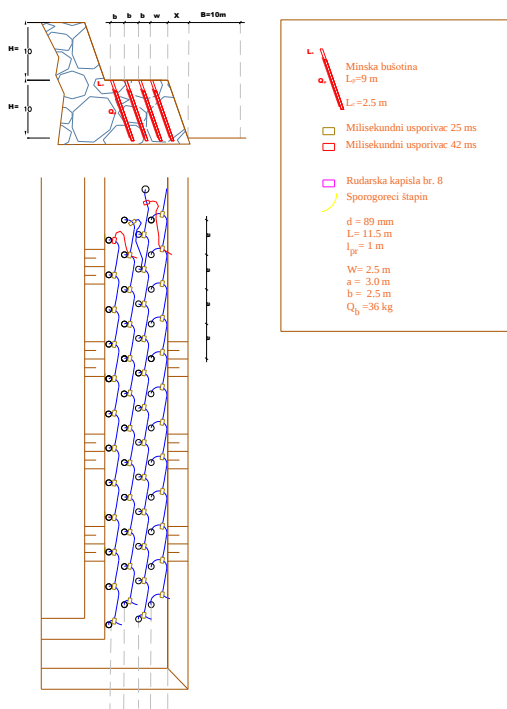
Slika 35. Višeredna šema Iniciranja minskih bušotina Nonel sistemom
