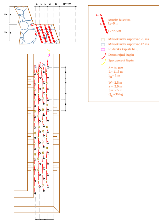
Slika 34. Višeredna šema iniciranja minskih bušotina det. štapin-udarna patrona
