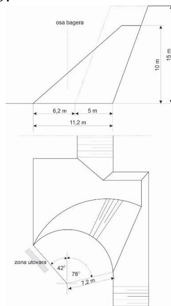
Slika 38. Tehnološka šema rada bagera
