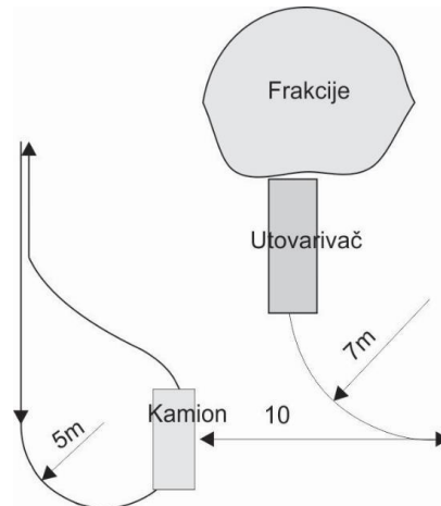
Slika 40. Tehnološka šema rada utovarača
