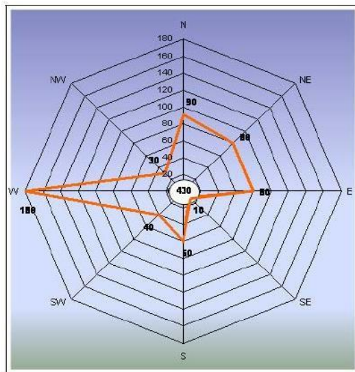
Sl.27. Klimatološka ruža
