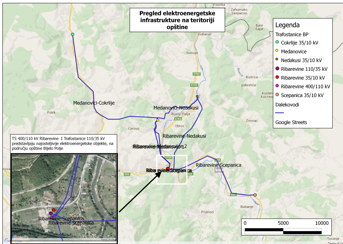
Gis mapa br. 3 pregled osnovne elektroenergetske infrastrukture
